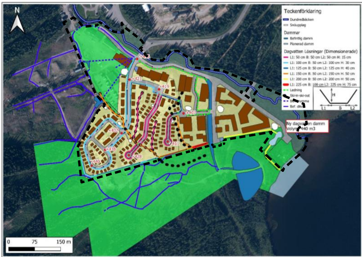
Figur 33. Dundret Gällivare Fjällanläggning AB:s systemlösning för dagvattenhantering. Anlagda dammar, sedimenteringsstråk och diken i mörkblått, föreslagen ny damm för omhändertagande av dagvatten från det östra området i ljusblått (AFRY, 2024). Uppdaterad planområdesgräns streckad svart linje.
