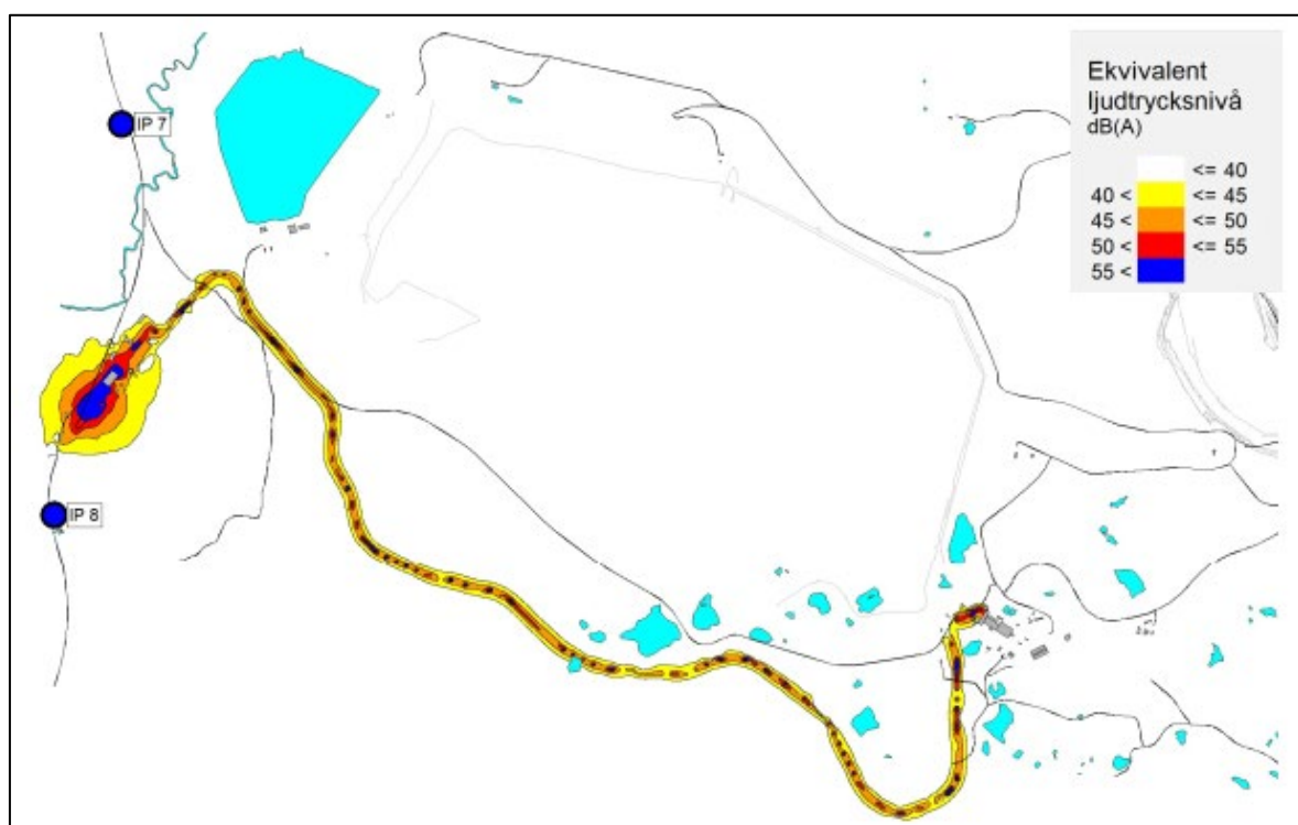
Figur 23. Beräknade ekvivalenta nivåer från nya bangården.
