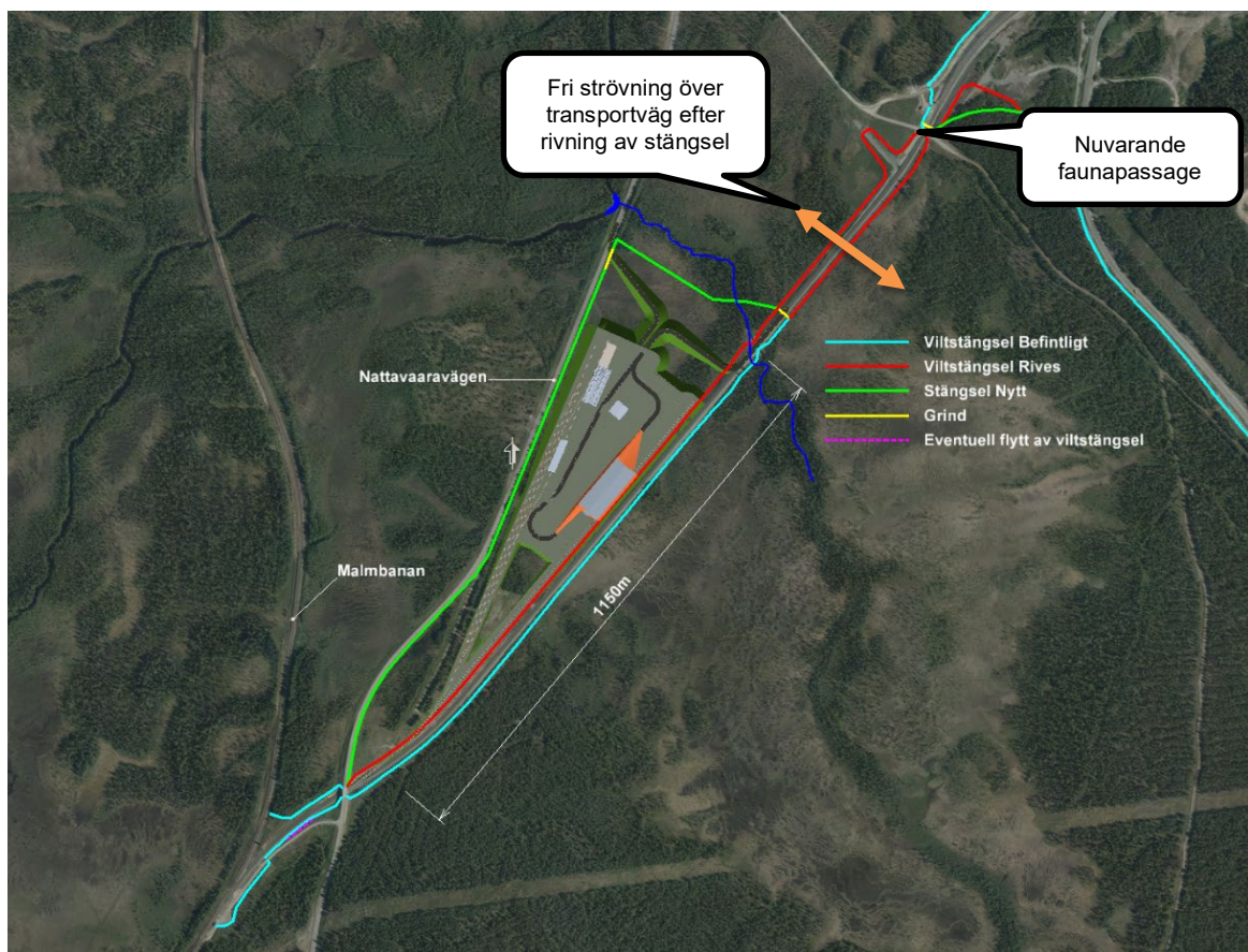
Figur 12. Befintligt och nytt viltstängsel.
