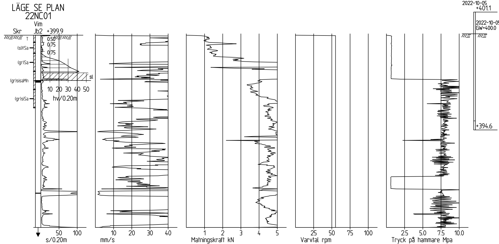
SONDERINGSRESULTAT 1:100
