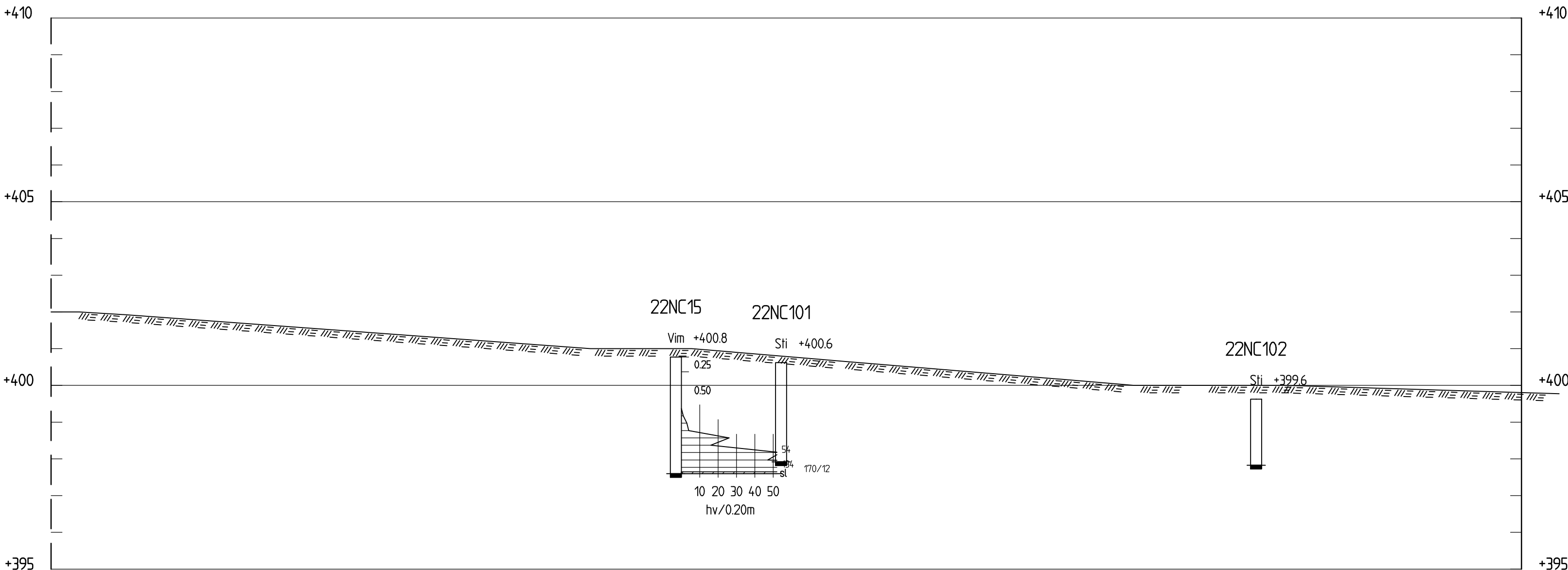
SEKTION C-C FORT. H 1:100 L 1:200
