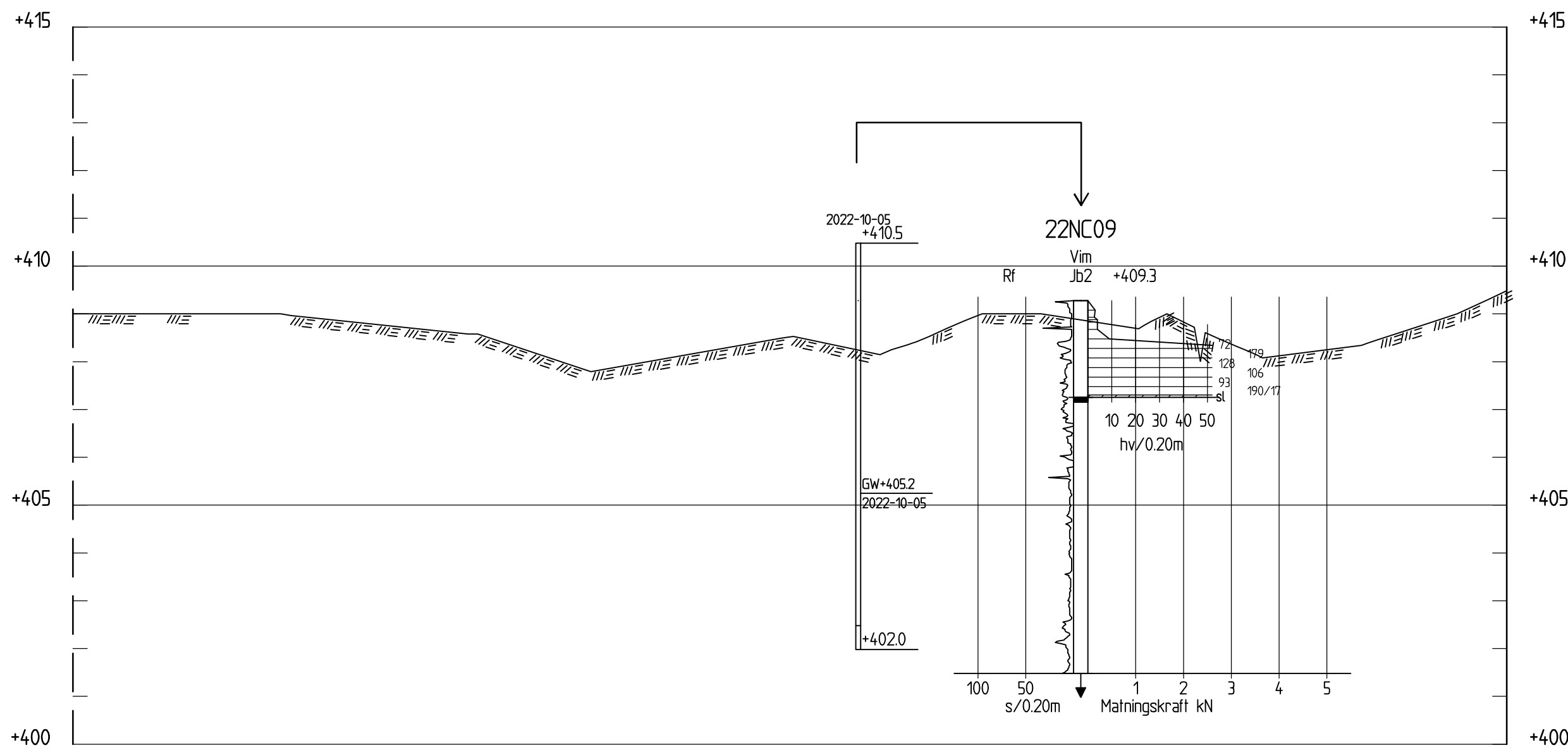
SEKTIÖN H-H FORT. H 1:100 L 1:200
