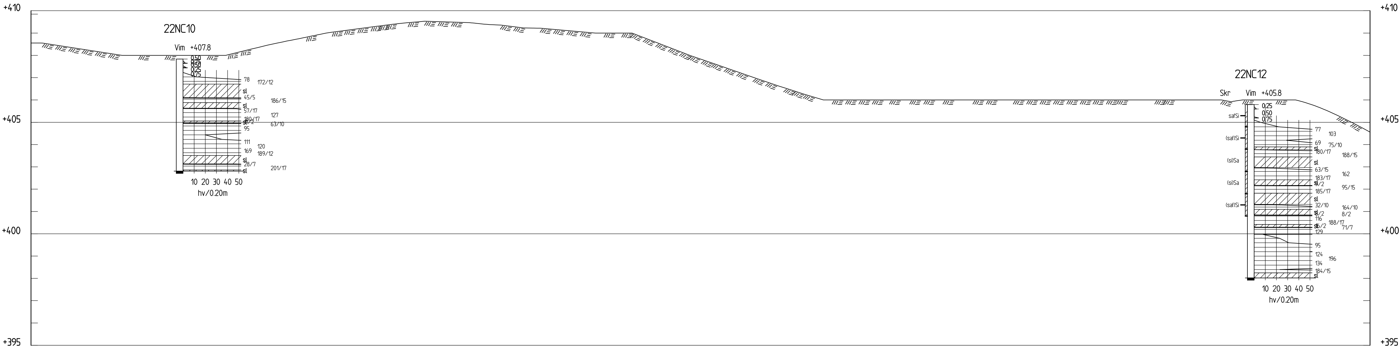
SEKTION D-D H 1:100 L 1:200
