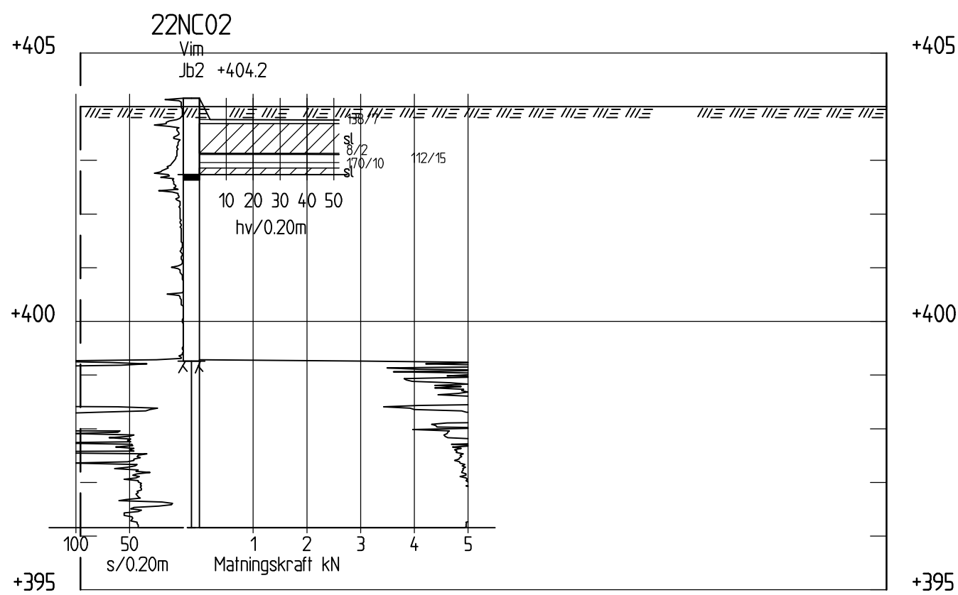
SEKTION J-J FORT. H 1: 100 L 1: 200
